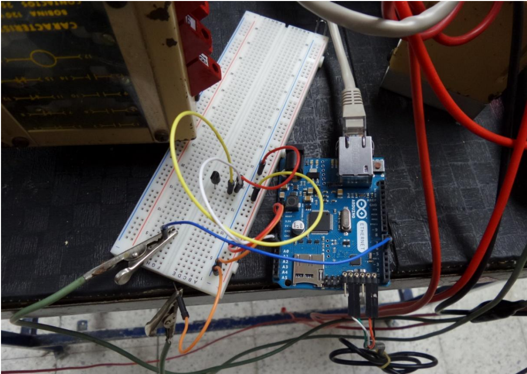
Fig. 3.20 Conexión arduino- protoboard y sensores.
