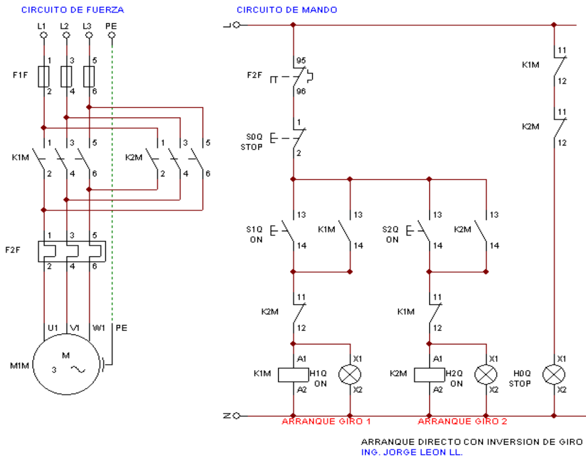
.Fig. 3.8 Circuito de potencia y control.
