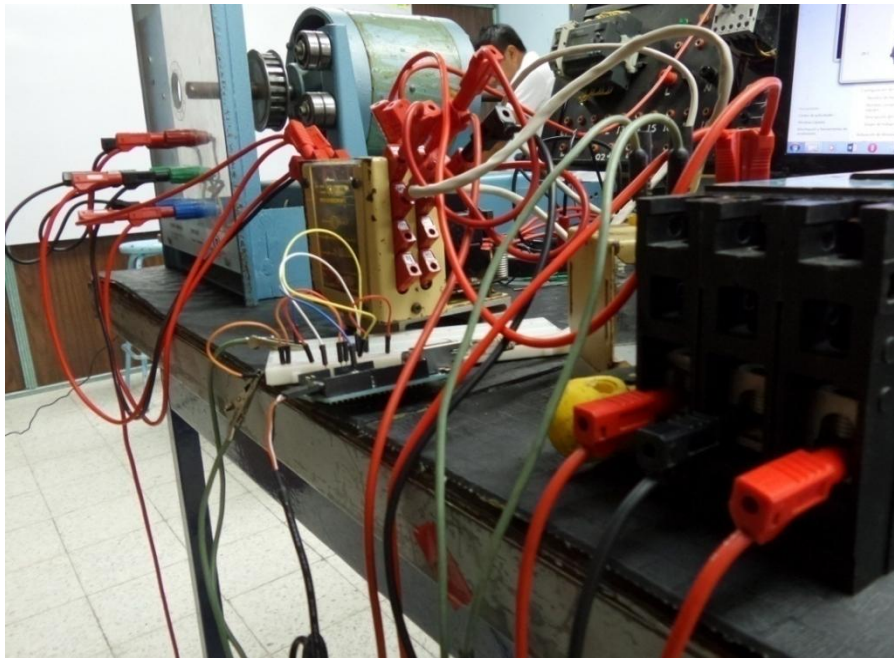
Fig. 3.21 Conexión de todo el sistema.
