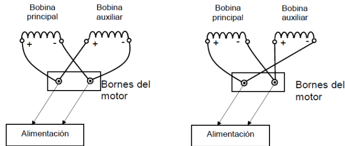
Fig. 3.7 Esquema para realizar el cambio del sentido de giro de un motor monofásico.
