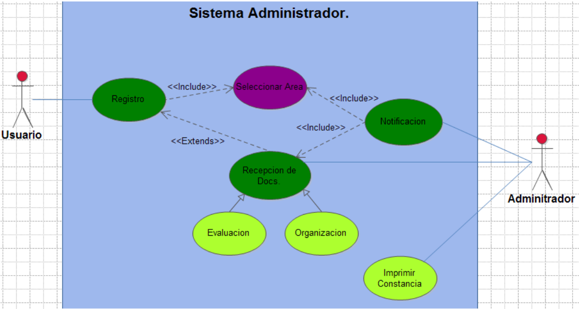
Figura 9.2. Diagrama de casos de uso de la aplicación.
