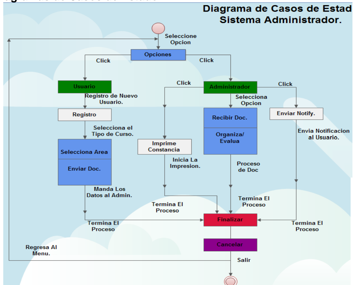
Figura 9.5. Diagrama de casos
