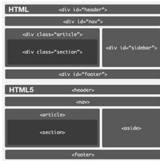
Figura 7.1. Estructura de HTML5. [2]
