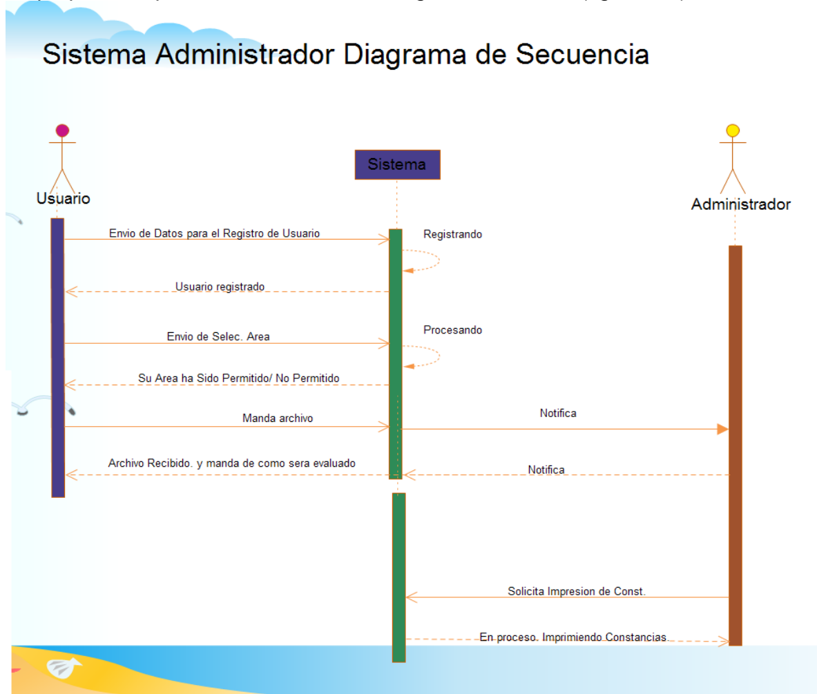
Figura 9.1. Diagrama de bloques de secuencia de la interfaz.
