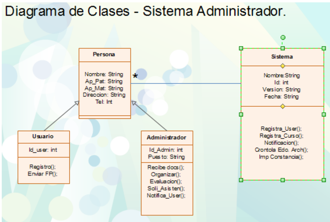
Figura 9.3. Diagrama de clases de la aplicación.
