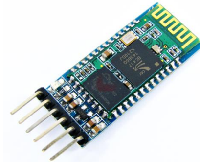
FIGURA 6.4 Módulo bluetooth con el que se establecerá la conexión con la tableta.
