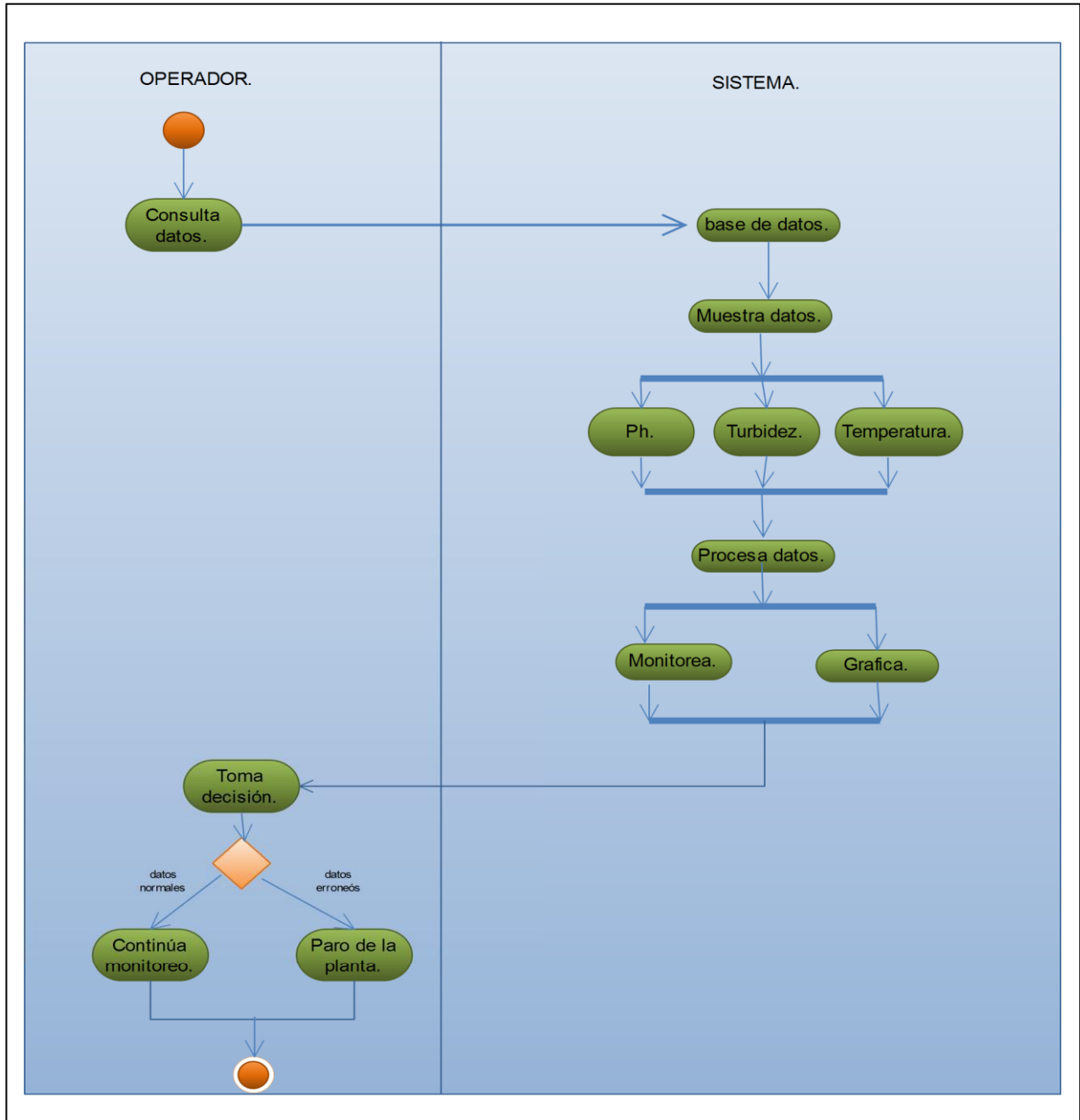
Fig. 17.- Diagrama de actividades.
