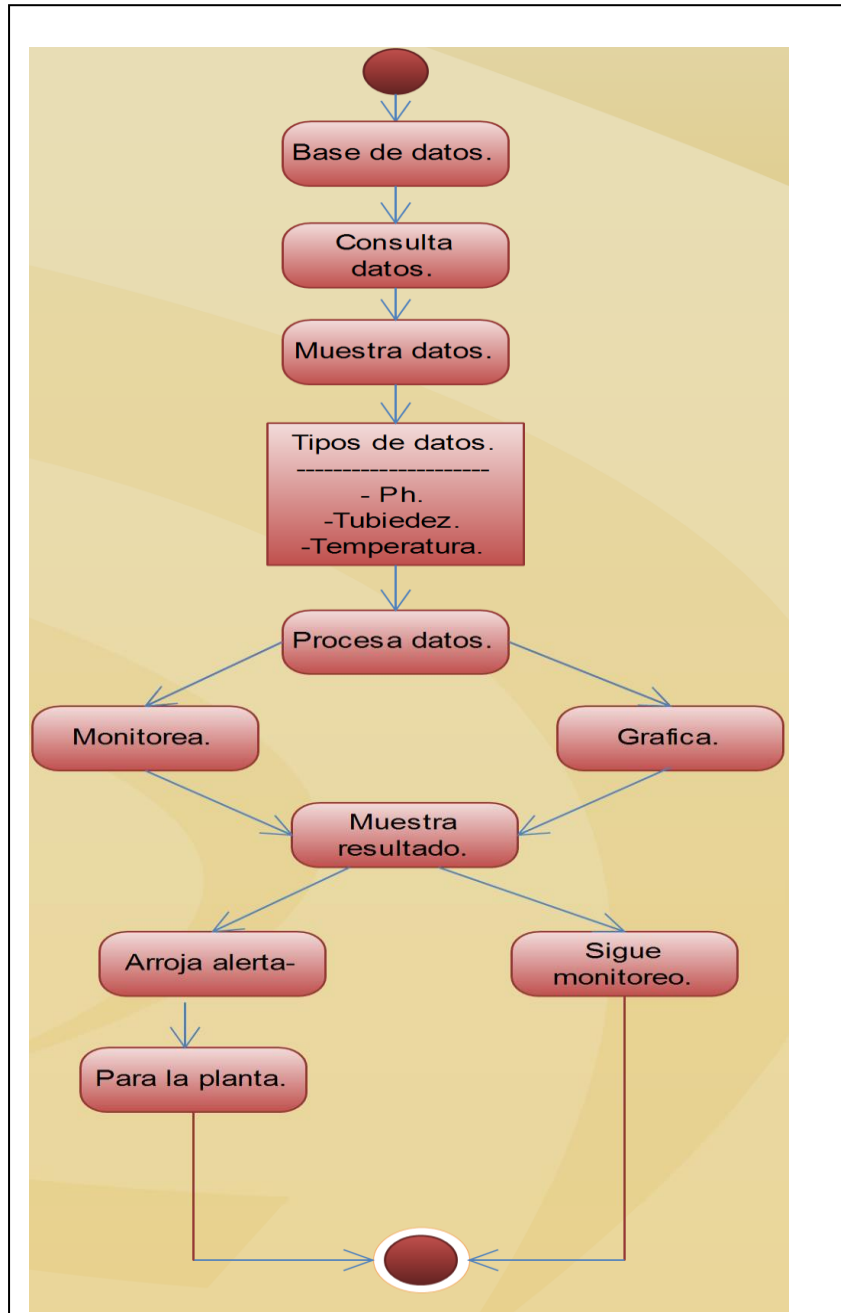
Fig. 15.- Diagrama de estados.
