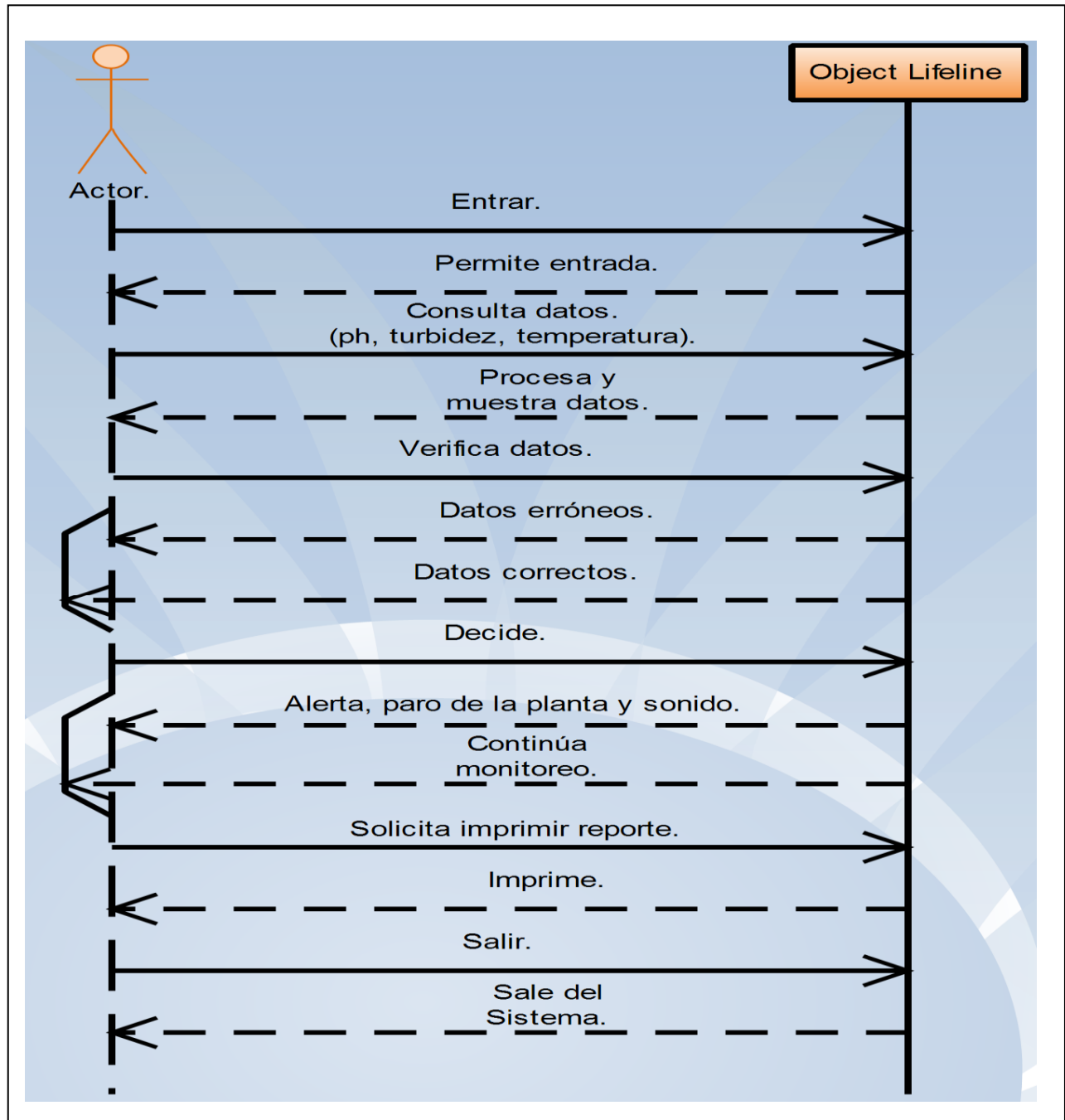
Fig. 16.- Diagrama de secuencia.
