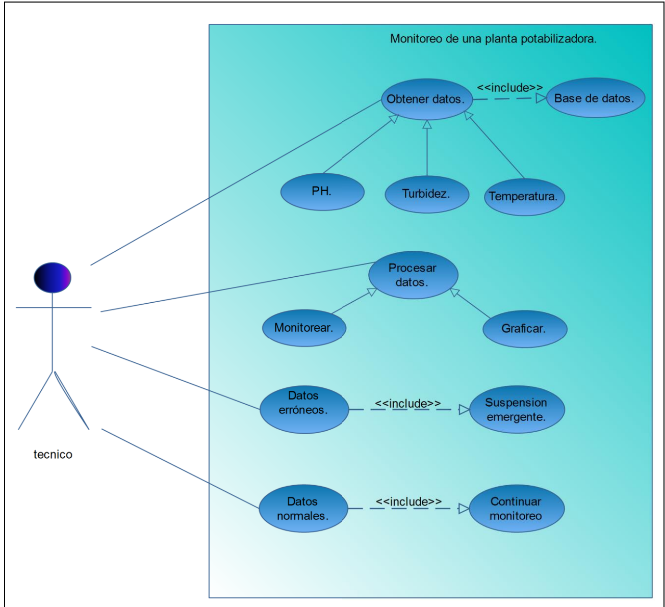
Fig. 14.- Casos de uso.
