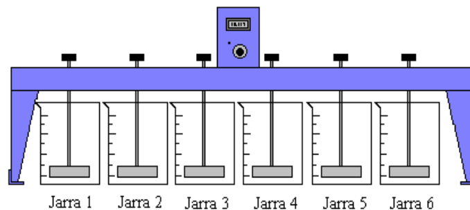
Fig. 10.- Prueba de jarras.
