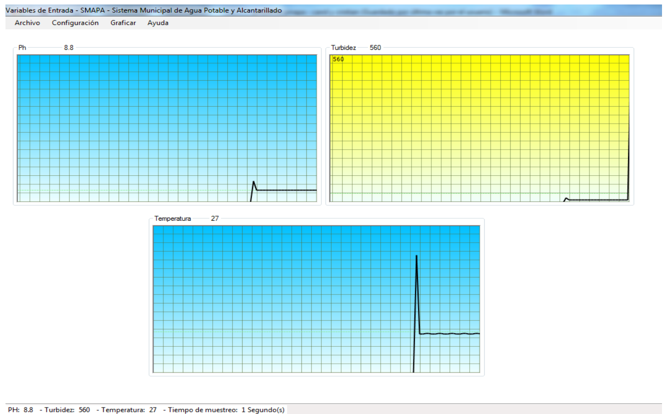
Fig. 23.- Alarma 1.
