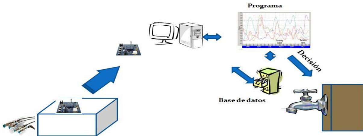
Fig. 31.- Diagrama gráfico.
