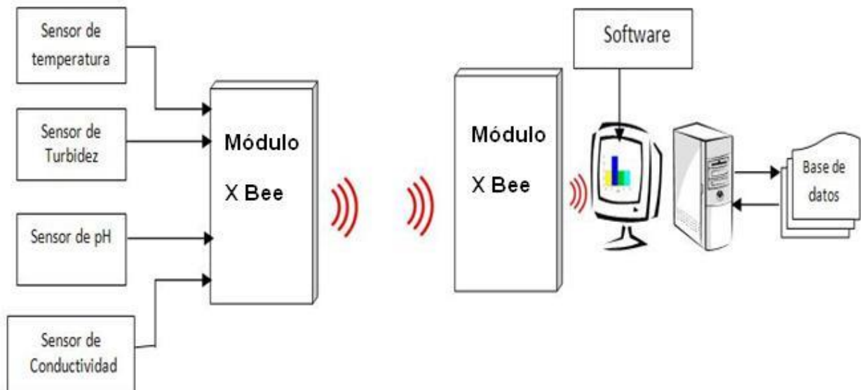
Fig. 28.- Diagrama a bloques general.
