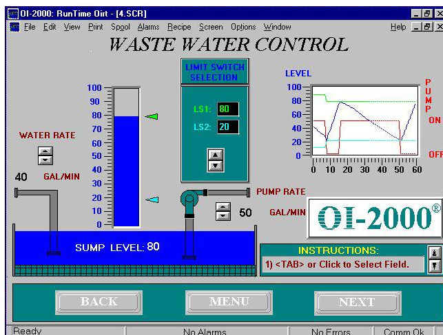
Fig. 5.- Pantalla principal de SCADA.
