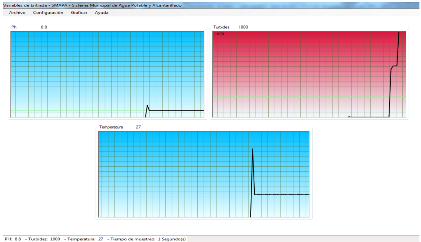
Fig. 24.- Alarma 2.
