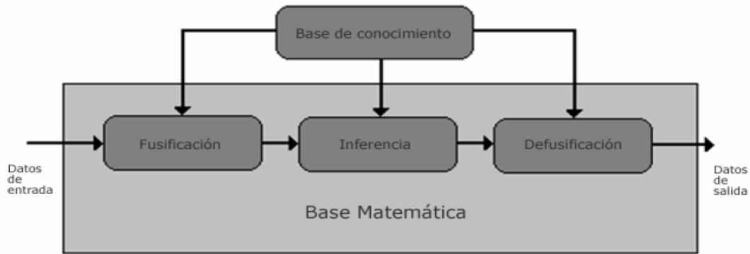
Fig. 30.- Lógica difusa.
