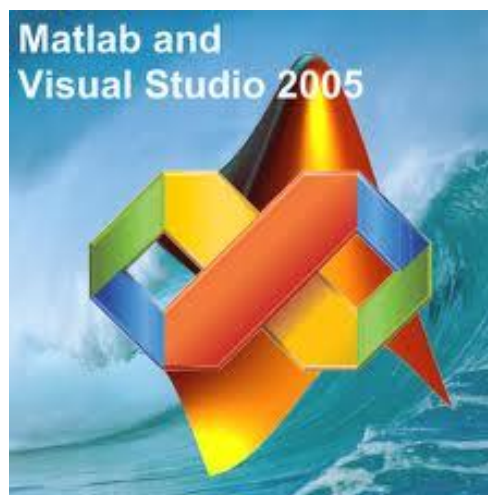
Fig. 12.- Visual studio.
