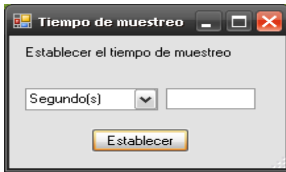
Fig. 26.- Establecer tiempo.
