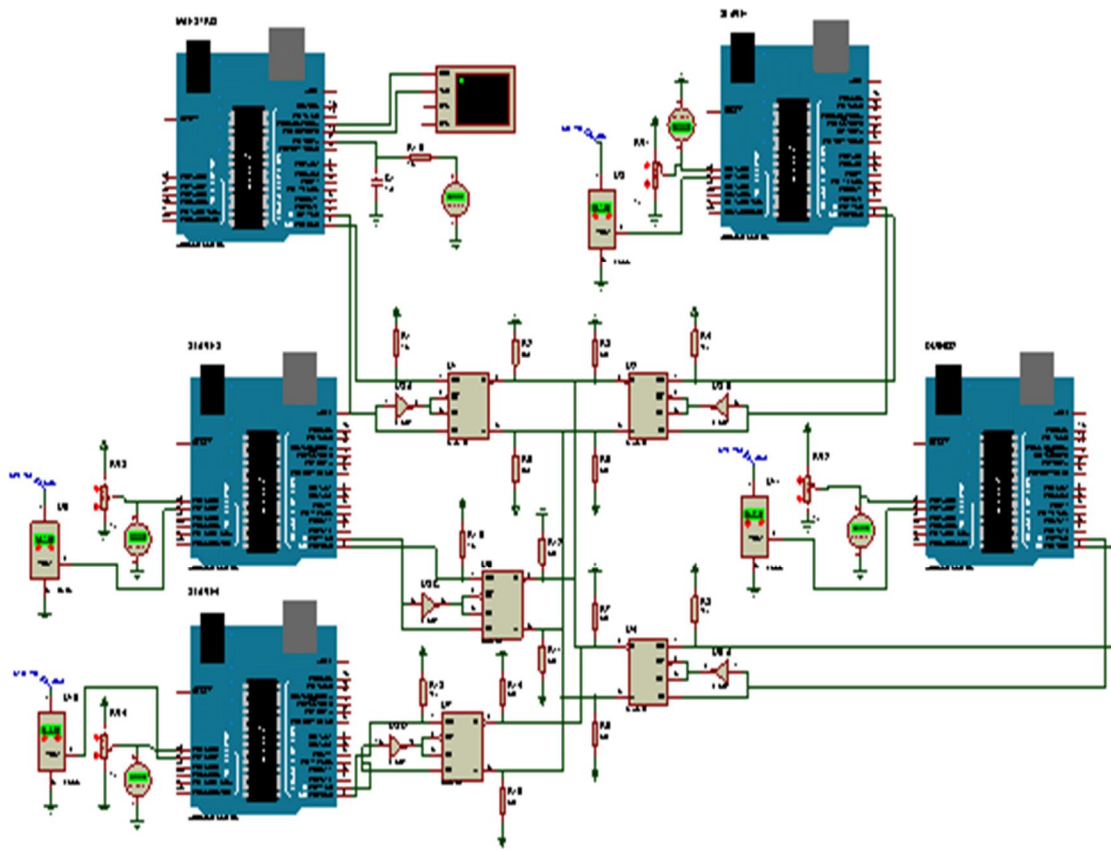
Figura 4.3: Comunicación con RS-485 entre Arduino maestro- esclavo
