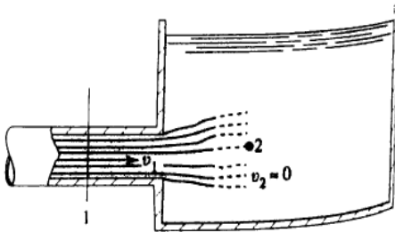
Fig. 3.9 Pérdida en la salida conforme el fluido pasa de una tubería a un depósito estático.
