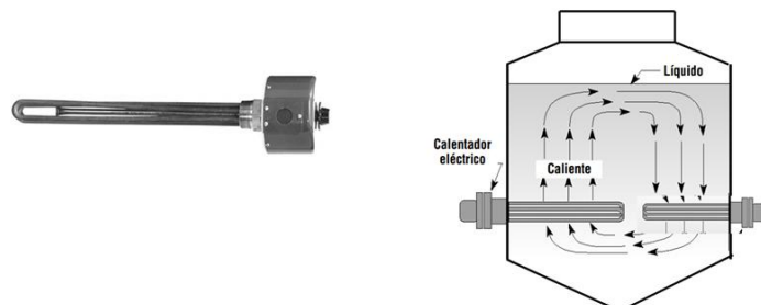
Fig. 4.7 Resistencia electrica propuesta
