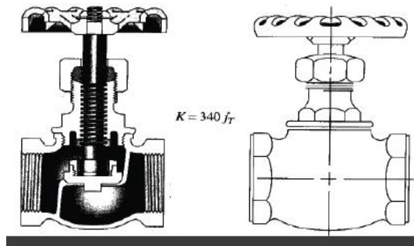
Fig. 3.5 Válvula de globo.
