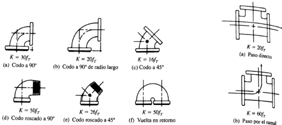
Fig. 3.8 Codos de tubería y Tes estándar.
