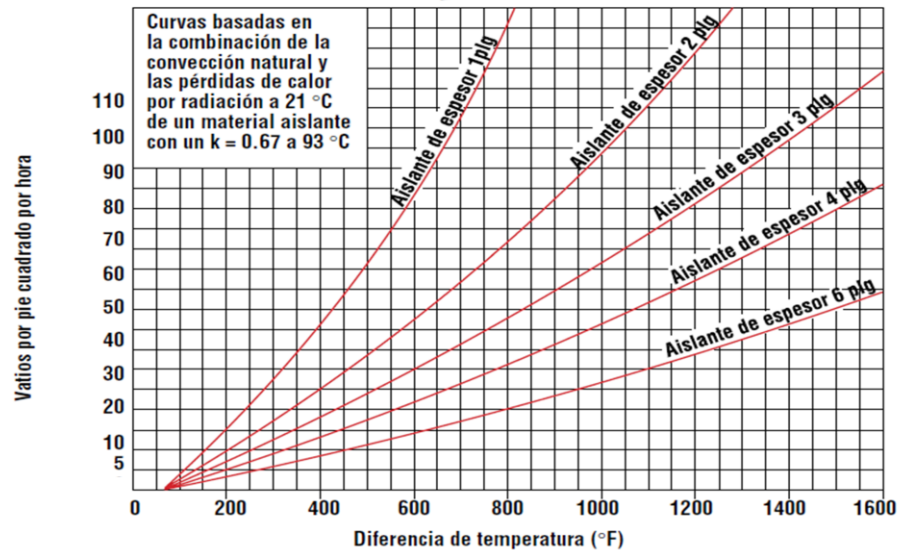
Gráfico G-126S: Pérdidas de calor de superficies de paredes aisladas de hornos, tuberías, tanques, etc.
