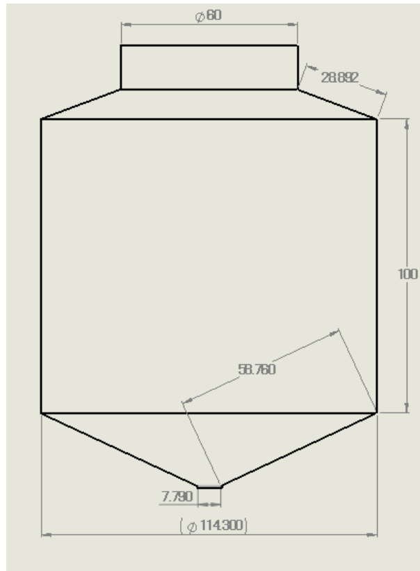
Fig. 4.6 Dimensiones del deposito.
