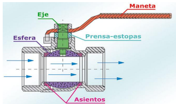
Fig. 3.7 Válvula de bola.
