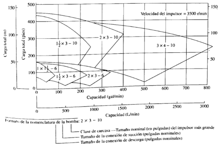
Fig. 3.13 Gráfica compuesta de rendimiento para una línea de bomba centrífuga.
