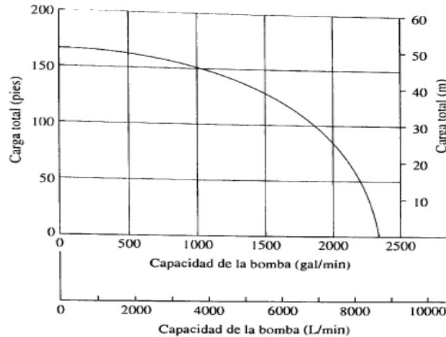
Fig. 3.12 Curva de rendimiento de una bomba centrífuga.
