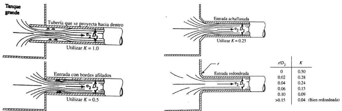
Fig. 3.10 Coeficiente de resistencias de entradas.
