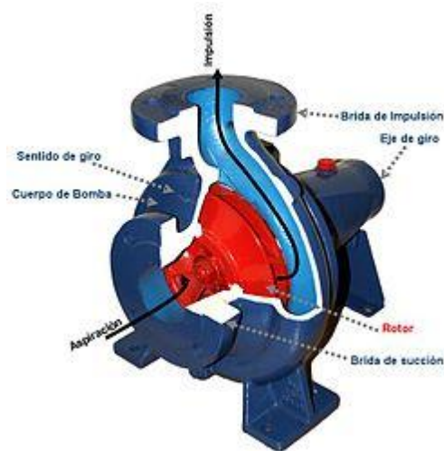
Fig. 3.11 Bomba centrífuga.
