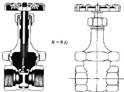
Fig. 3.6 Válvula de compuerta.
