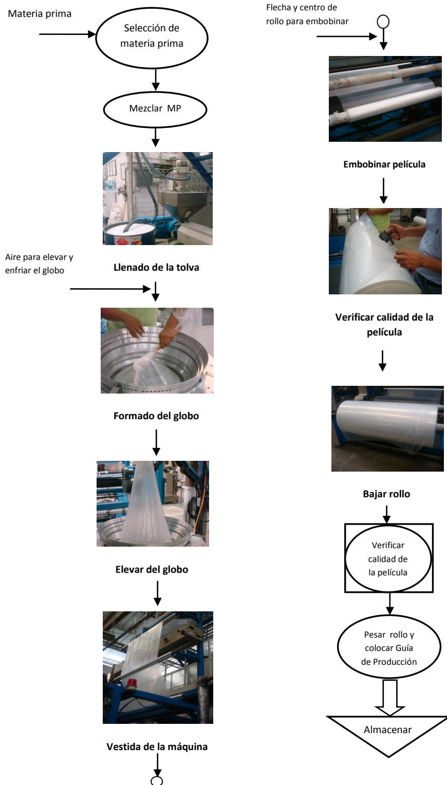
Figura 5.4 Diagrama de flujo del área de rollo punteado.
