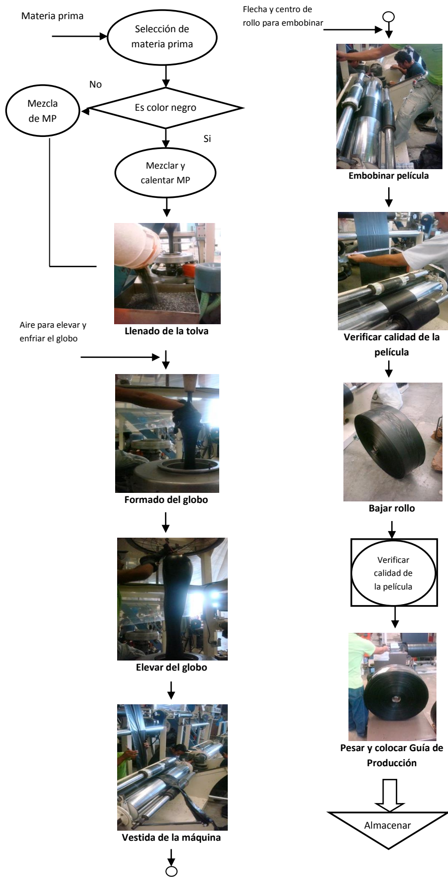
Figura 5.1 diagrama de flujo del área de camisetitas
