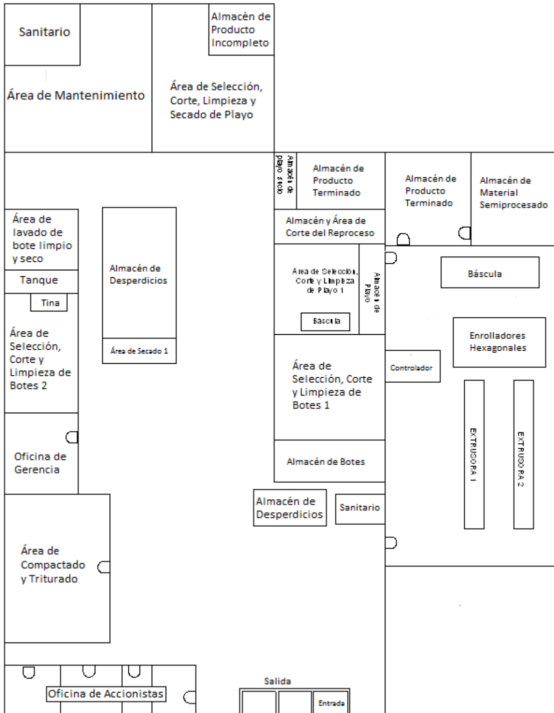
Figura 3.2 Distribución de la Planta 26.
