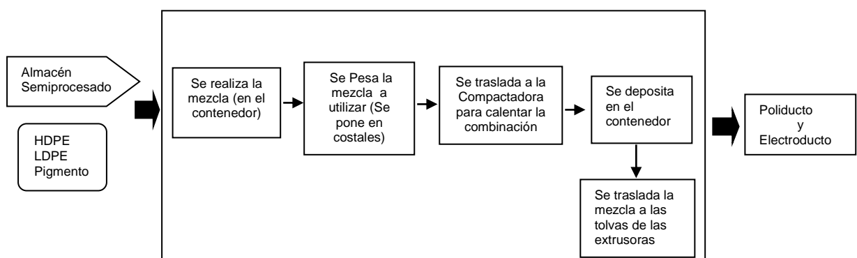
Figura 4.1 Proceso de Producción de Mangueras 31
