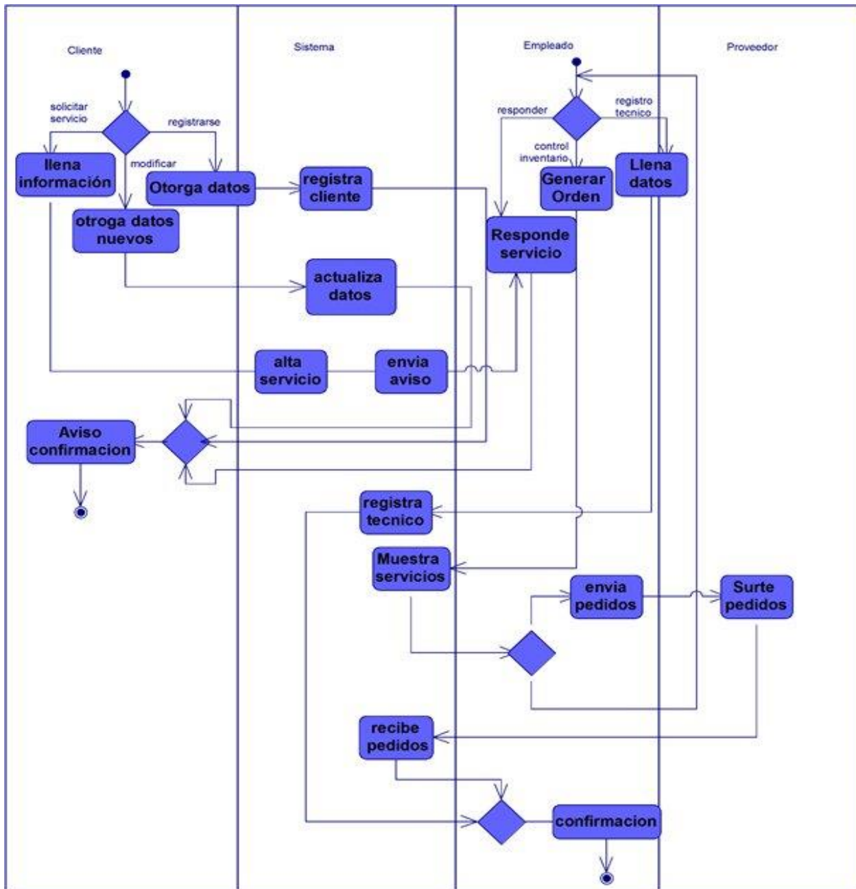
Fig.3 Diagrama de actividades.
