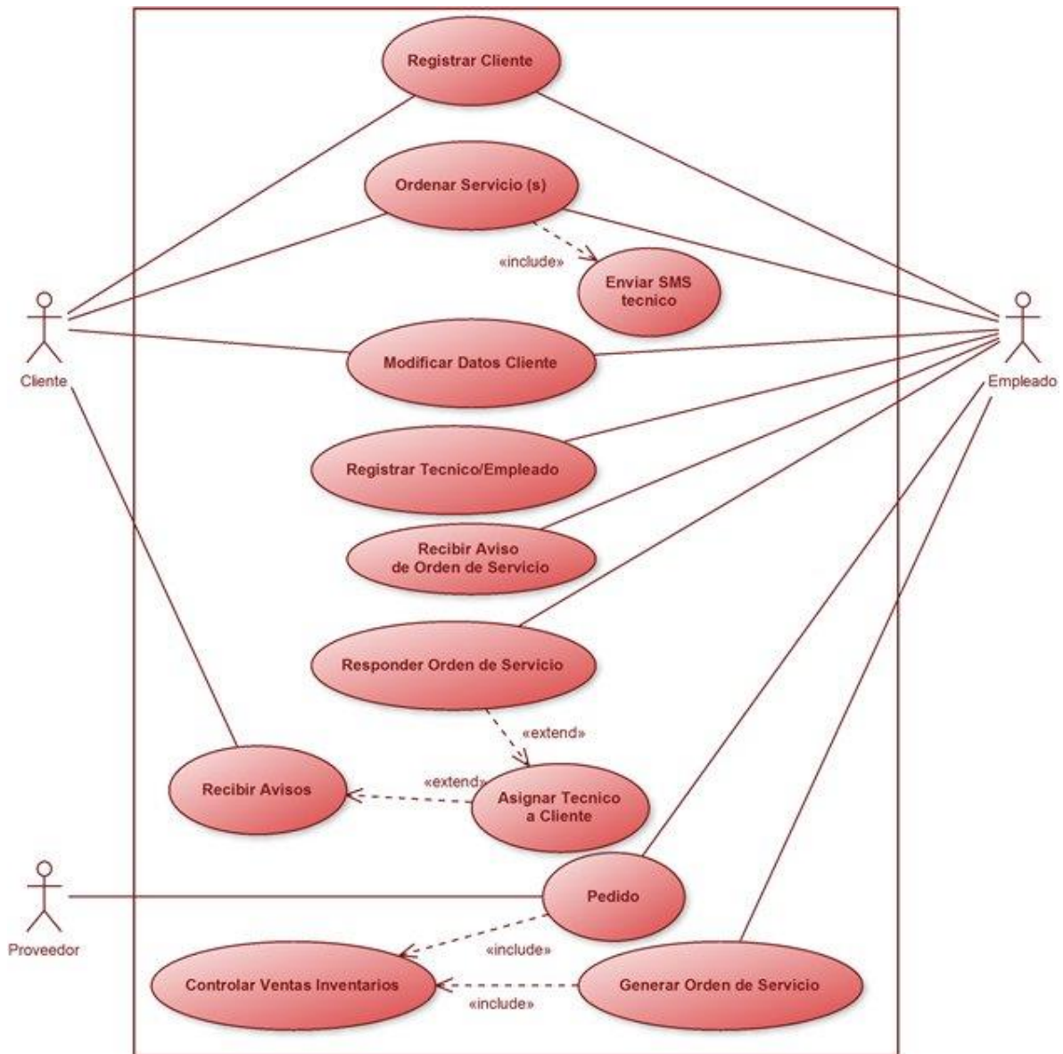
Fig.4 Diagrama de casos de uso.
