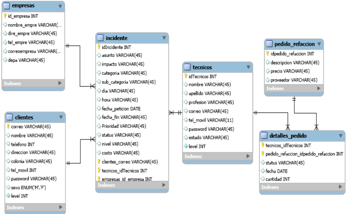
Fig.2 Base de datos relacional.
