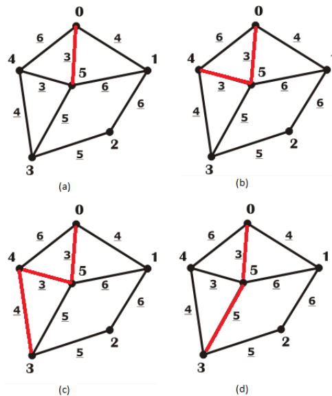
Fig. 9. Ejemplo de Dijkstra.
