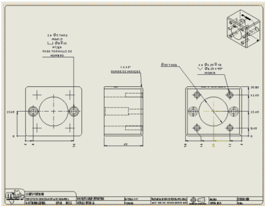
Plano dimensional de la pieza PM7RH – 26.
