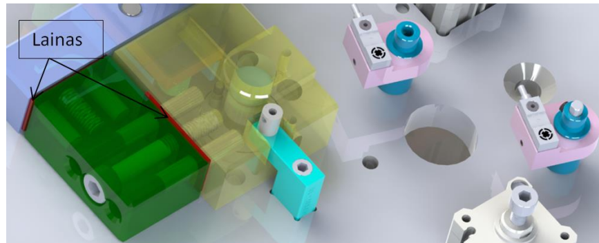
Figura 4.32. Laineo del sub-ensamble: "Base-Tubo".
