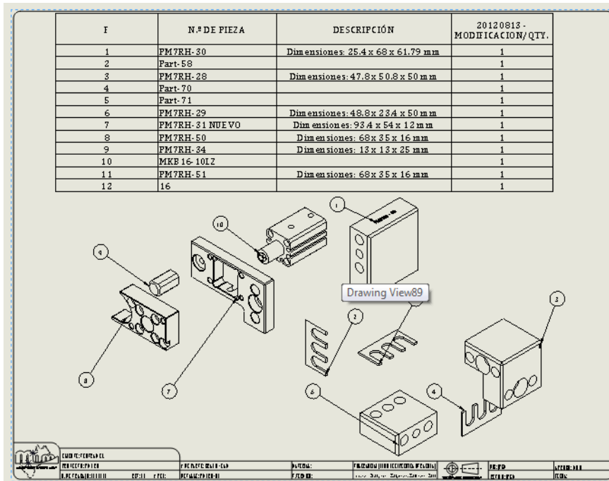
Plano dimensional del Subensamble Brazo-Cam.
