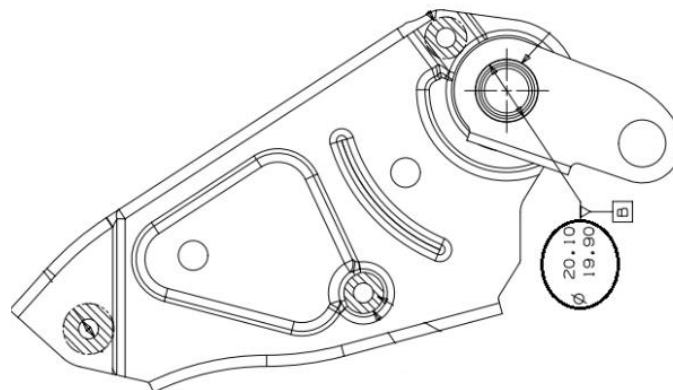
Imagen 4.28. Concentricidad del diametro del “Pive-tube” y “Cover-plate”.
