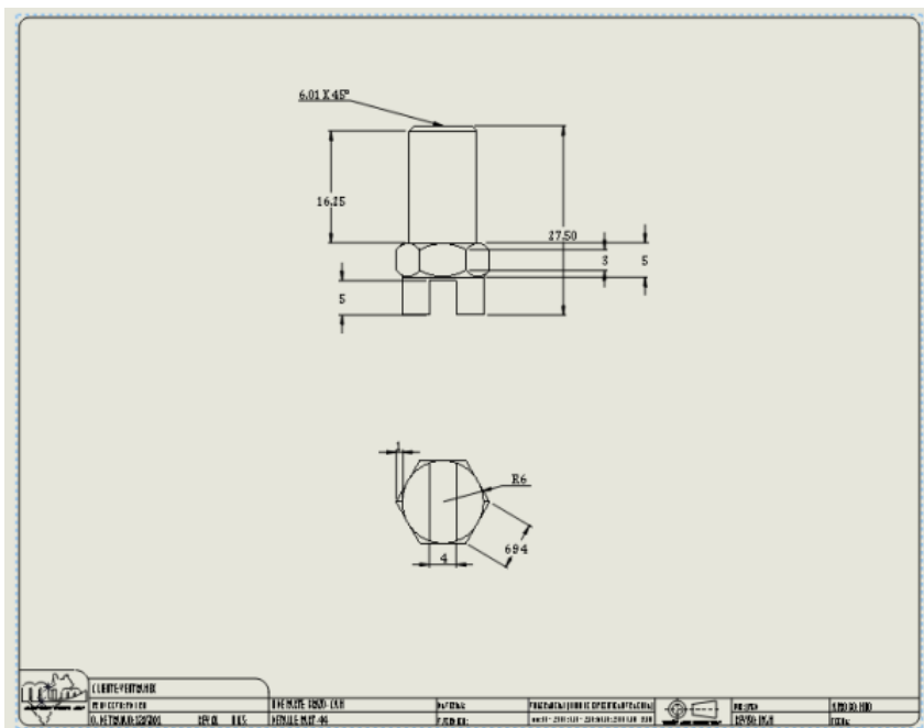
Plano dimensional de la PART – 44.
