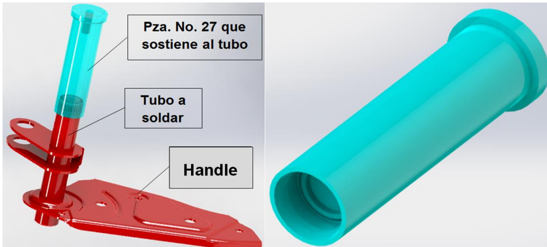
Figura 4.5. Diseño mejorado de la pieza PM7RH-27.
