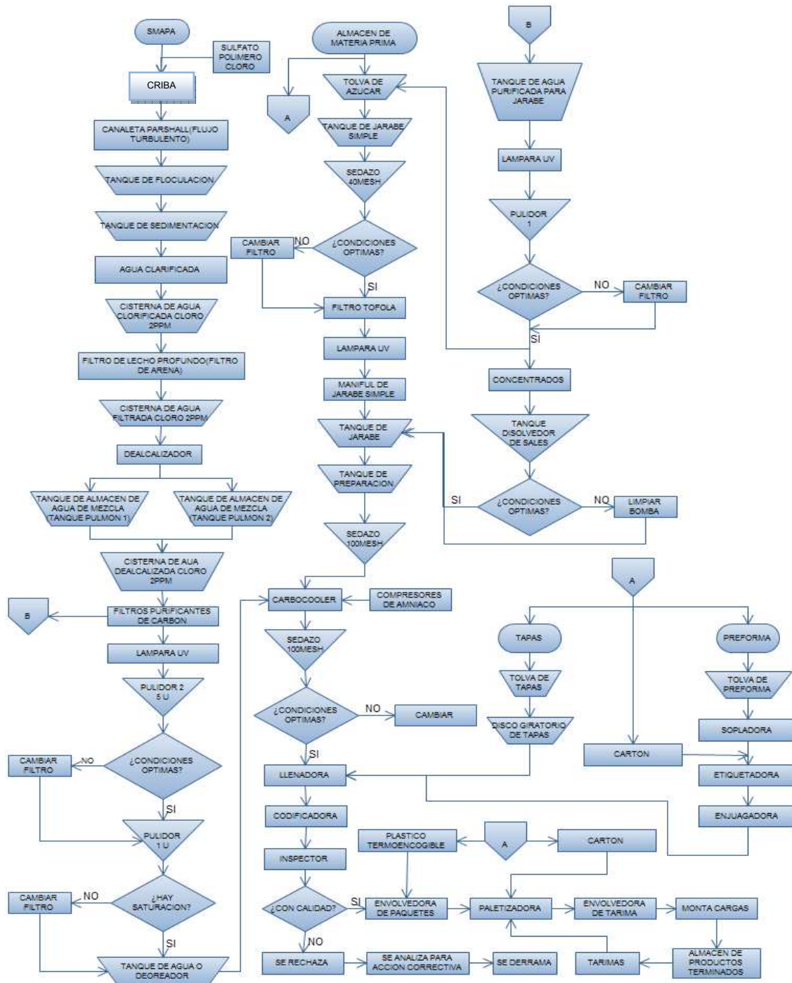
Fig. 2.3. Diagrama de flujo de los procesos productivos
