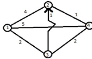
Fig. 10. Ejemplo Floyd-Warshall.
