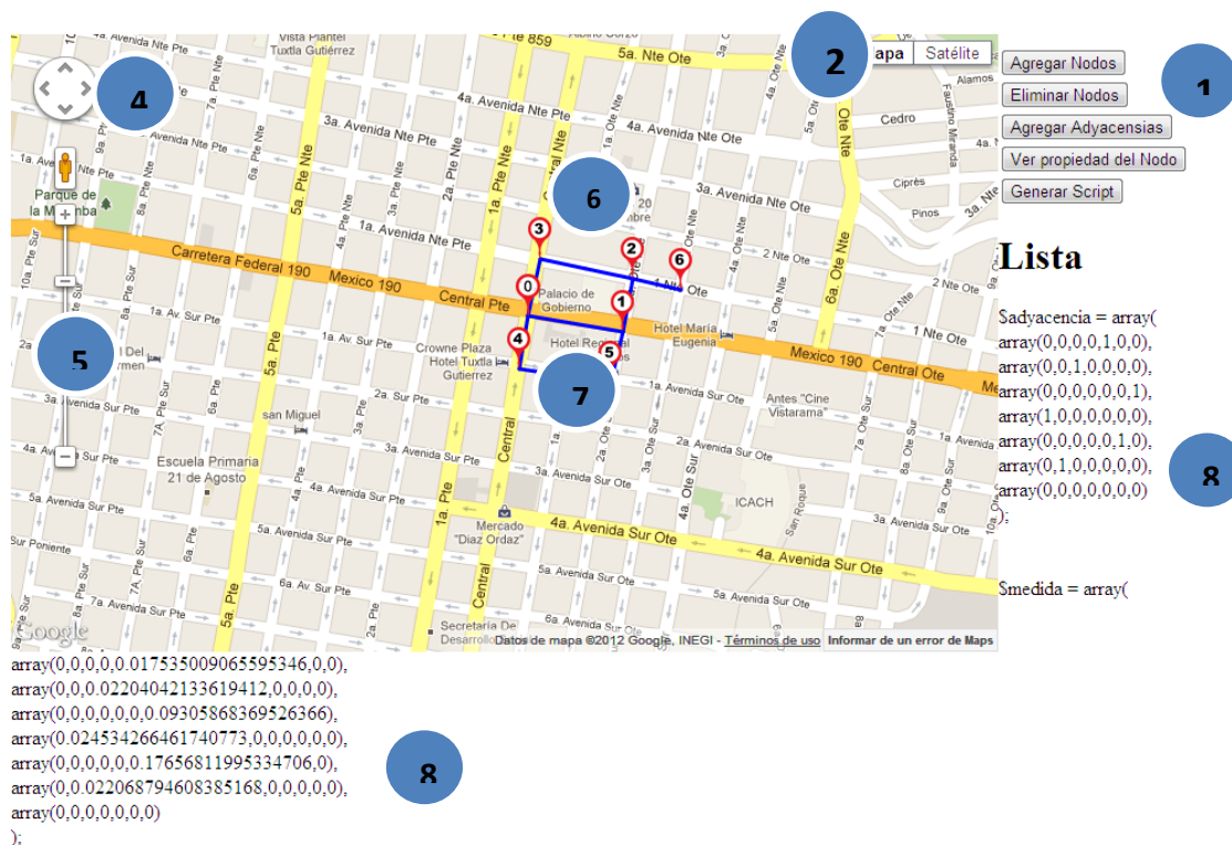
Fig. 24. Descripción del prototipo.
