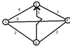
Fig. 10. Ejemplo Floyd-Warshall.
