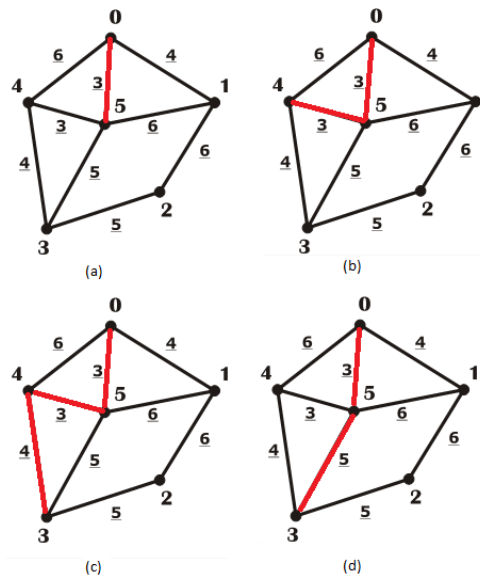
Fig. 9. Ejemplo de Dijkstra.
